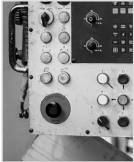
Ein altes Heidenhain-Bedienpult An early Heidenhain operator's panel
