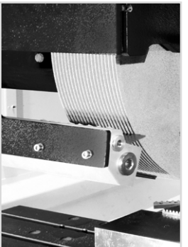
Automatische Kühlmittelzufuhrverstellung Track and follow coolant nozzles
