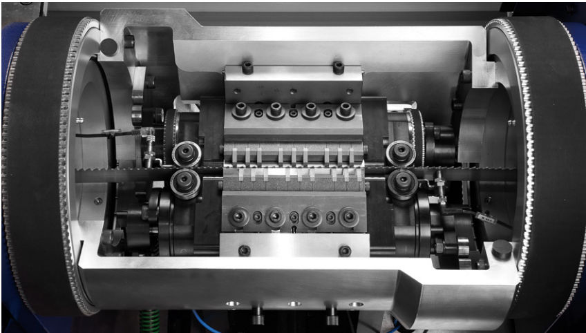
Baseline-Schränken – Das Kessel Schränkprinzip Baseline setting – The Kessel setting method
