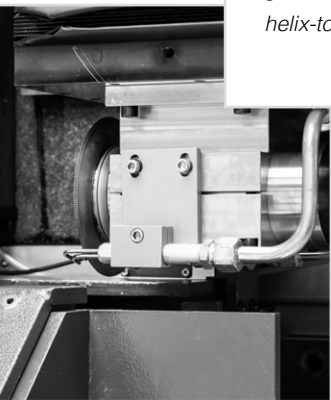
Abrichten mit Diamantformrand Dressing using a diamond wheel
